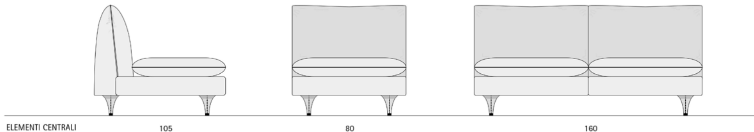
ELEMENTI CENTRALI
